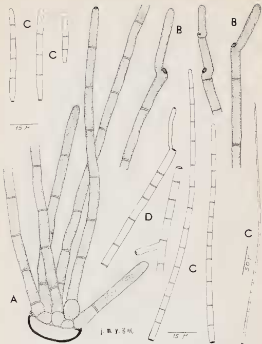
Fig. 3. — Cercospora lambareneensis Yen (nov. sp.): A, Fascicule de conidiophores ; B, Géniculations des conidiophores ; C, Conidies ; D, Germination des conidies.
